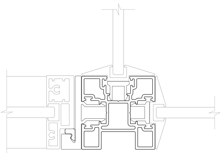
Nodo 3 vie con porta battente / 3 ways joint with swing door
