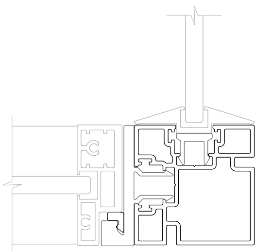
Nodo 2 vie con porta battente / 2 ways joint with swing door
